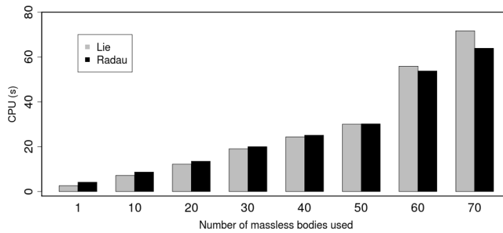
FIG. 3.2 – Temps CPU de calcul pour les intégrateurs de Lie (■) et Radau (■). L'axe des abscisses représente le nombre de petits corps intégrés simultanément.
