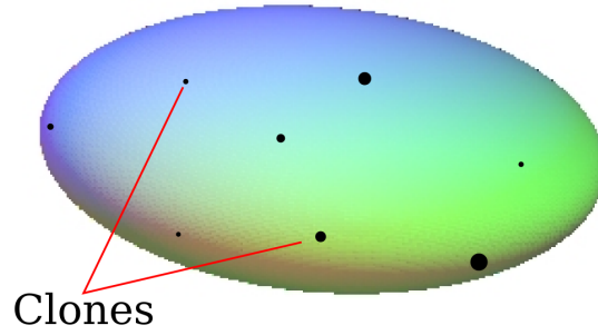
FIG. 5.4 – Ellipsoïde de confiance. Les points en noir représente les clones obtenus par une méthode d'échantillonnage.
