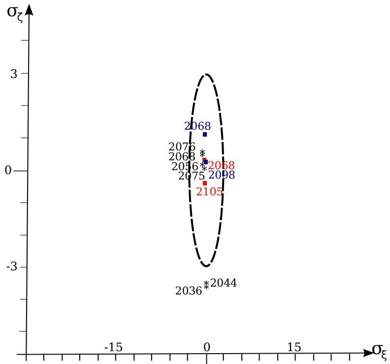
FIG. 5.10 – Zone d’incertiude à (\sigma_{\xi}, \sigma_{\zeta}) en 2029. La figure est centrée sur la valeur nominale (\xi, \zeta) . La position de keyholes primaires ( \star ) et de keyholes secondaires dont les impacts avec la Terre se situent au nœud ascendant (■) ou au nœud descendant (■) sont aussi indiquées.
