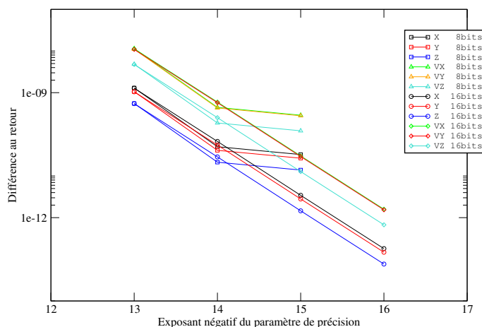
FIG. 4.2: Comparaison des méthodes d'intégration pour différentes valeurs du paramètre de précision \epsilon . Pour un calcul en double précision on peut voir très clairement un palier sur la précision du modèle. Ceci est dû à la limite de précision \epsilon_{machine} des calculs en double précision.
