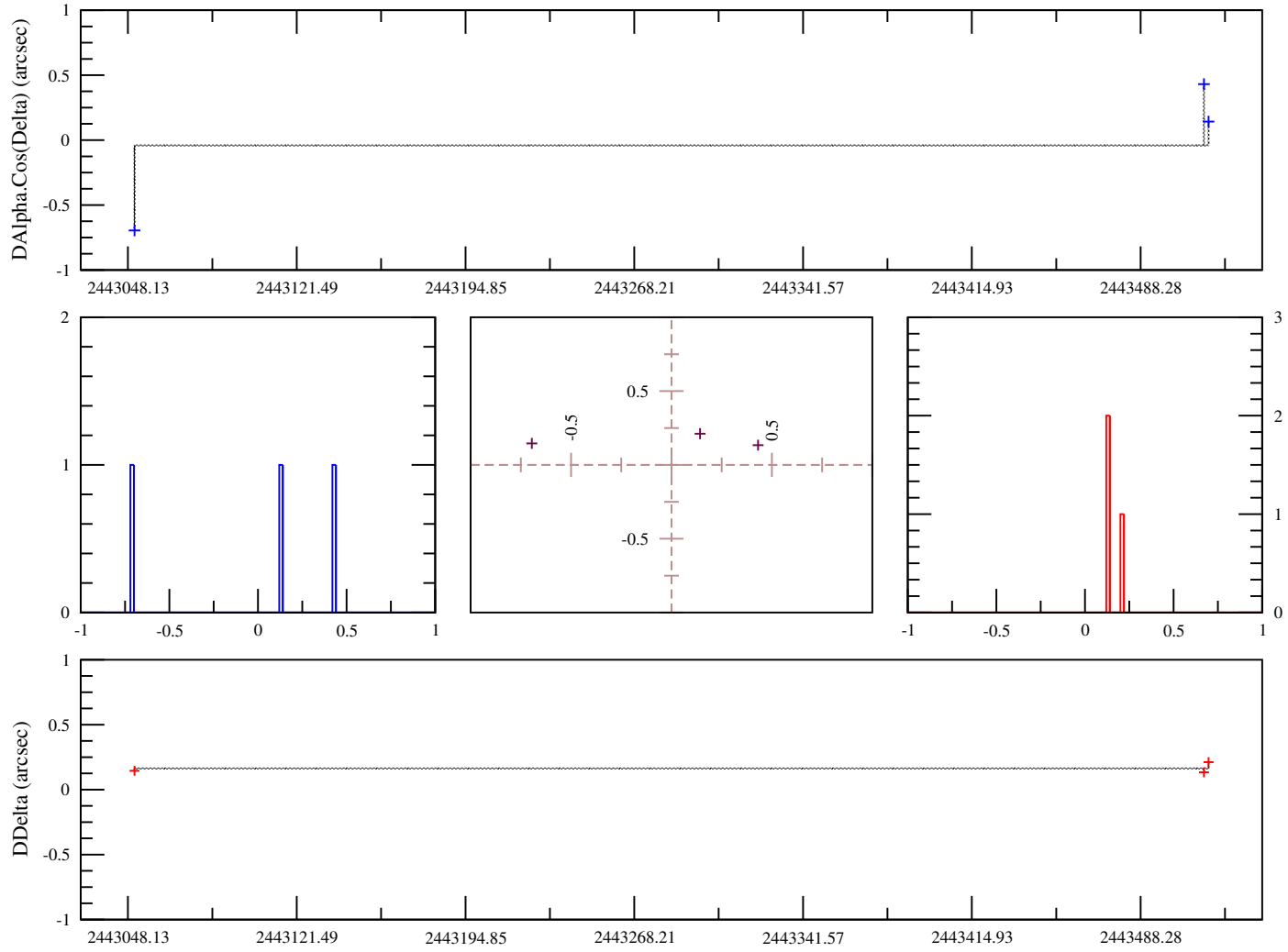
FIG. B.28: Observations Mulholland, 1977, Obs. McDonald, USA. OmC sur les observations d'Amalthee calculés avec l'éphéméride du JPL
