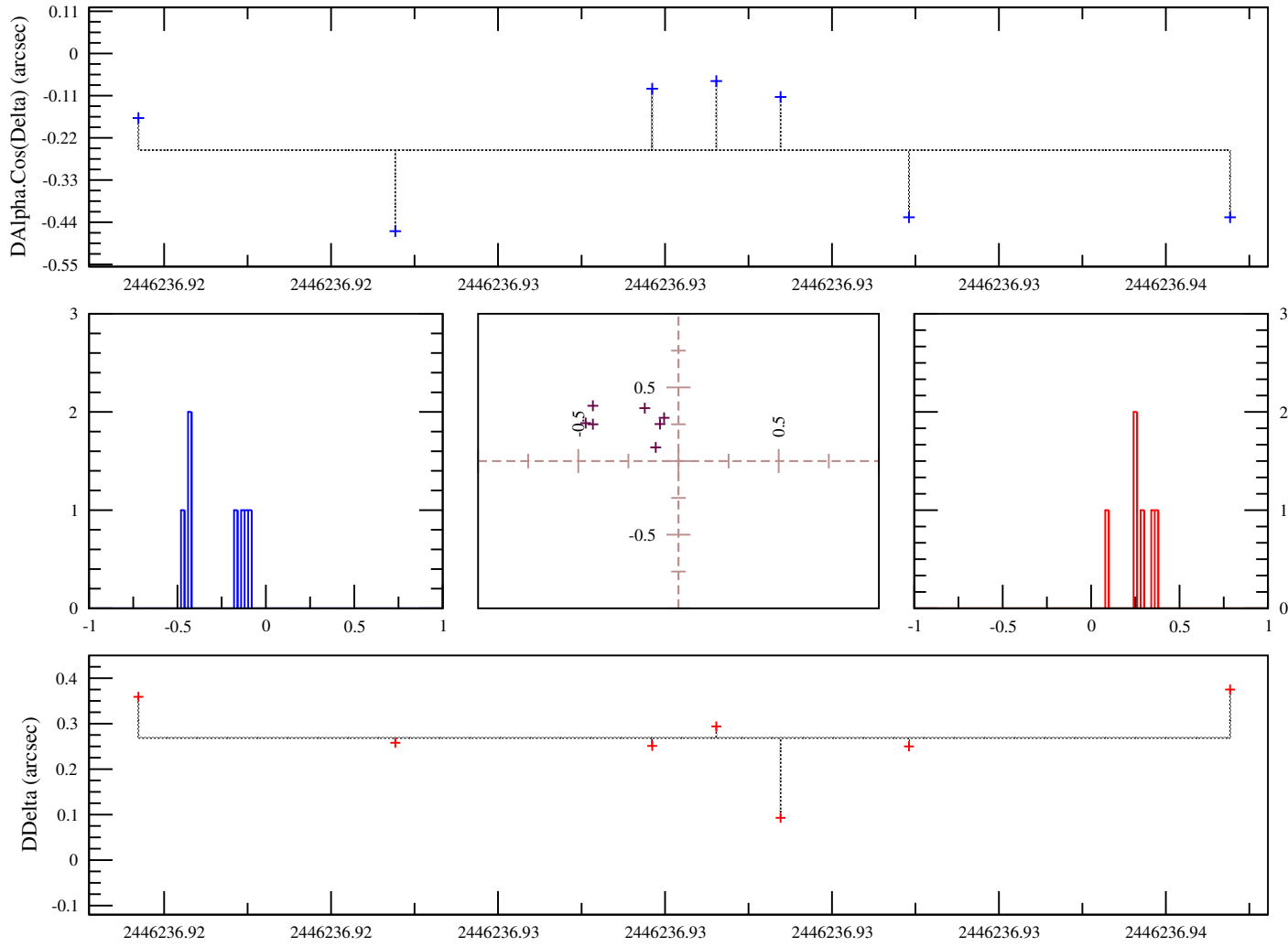
FIG. B.8: Observations Pasco D., 1985, USNO-Flagstaff, USA. OmC sur les observations de Thébé calculés avec l'éphéméride du JPL
