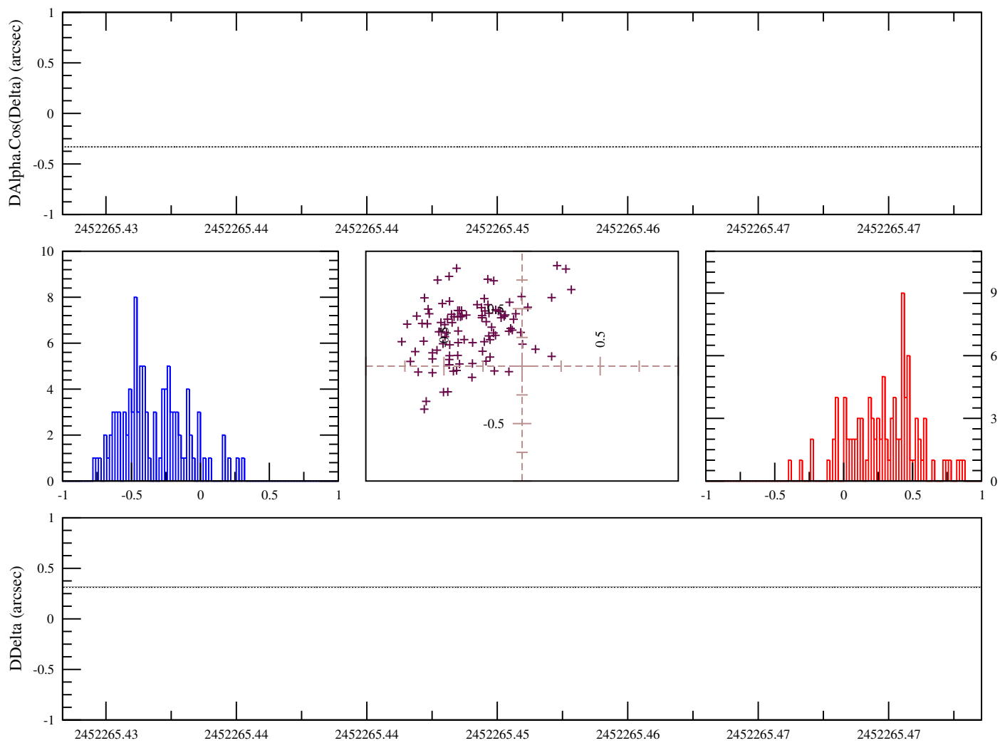
FIG. B.4: Observations Colas F., Vachier F., 2001, Pic du Midi, France. OmC sur les observations de Thébé calculées avec l'éphéméride du JPL
