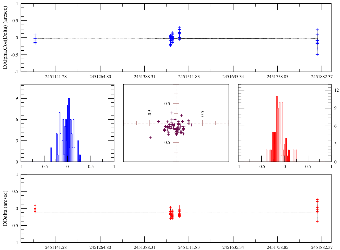
FIG. B.29: Observations Kulyk et al., 1998-2000, Pik Terskol, Ukraine. OmC sur les observations d'Amalthee calculées avec l'éphéméride NJO2004A
