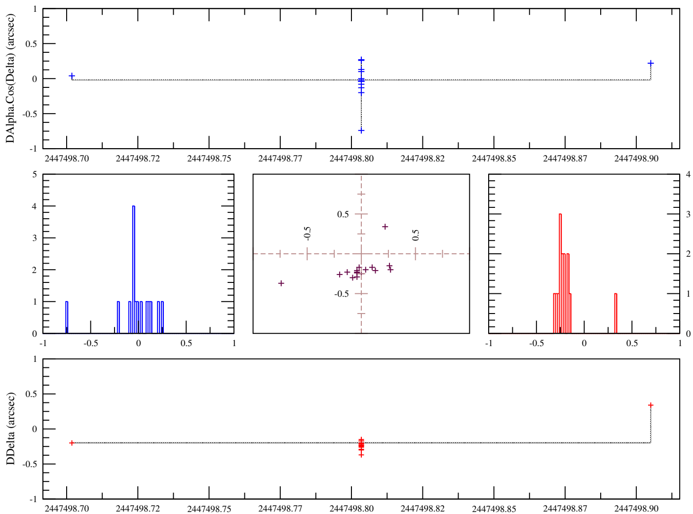
FIG. B.18: Observations Nicholson, 1991, Mt Palomar USA. OmC sur les observations d'Amalthée calculés avec l'éphéméride du JPL
