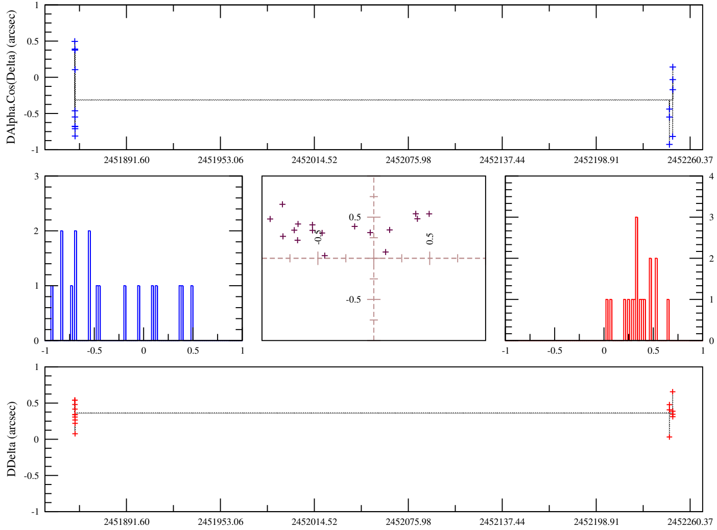
FIG. B.11: Observations Pasco D., Vachier F., 2001, USNO-Flagstaff, USA. OmC sur les observations de Thébé calculés avec l'éphéméride du JPL
