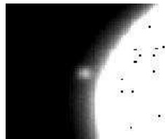
FIG. 2.2: Si on change les seuils de l'image on peut voir Amalthée qui se trouve à moins de 5" du bord de Jupiter.
