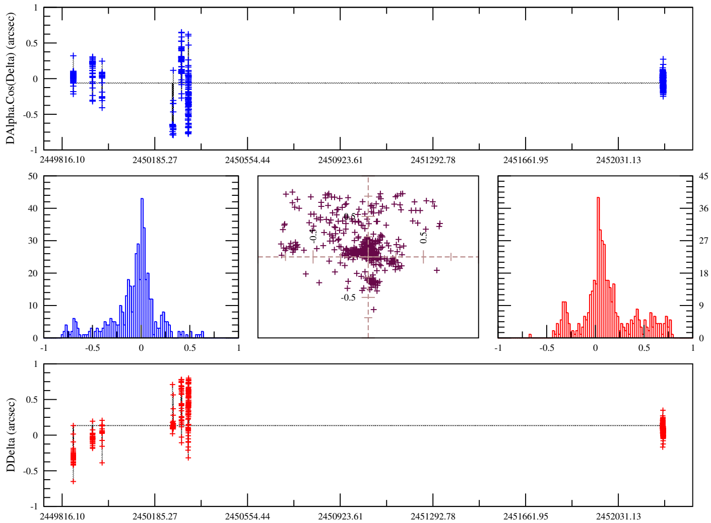
FIG. B.15: Observations Veiga C., Vieira-Martins R., 1995-2001, LNA Itajuba Brasil. OmC sur les observations d'Amalthee calculés avec l'éphéméride NJO2004A
