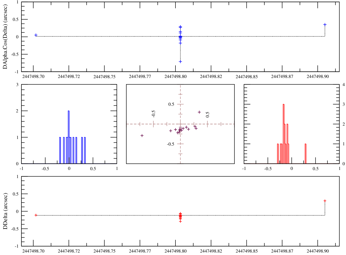
FIG. B.17: Observations Nicholson, 1991, Mt Palomar USA. OmC sur les observations d'Amalthée calculés avec l'éphéméride NJO2004A
