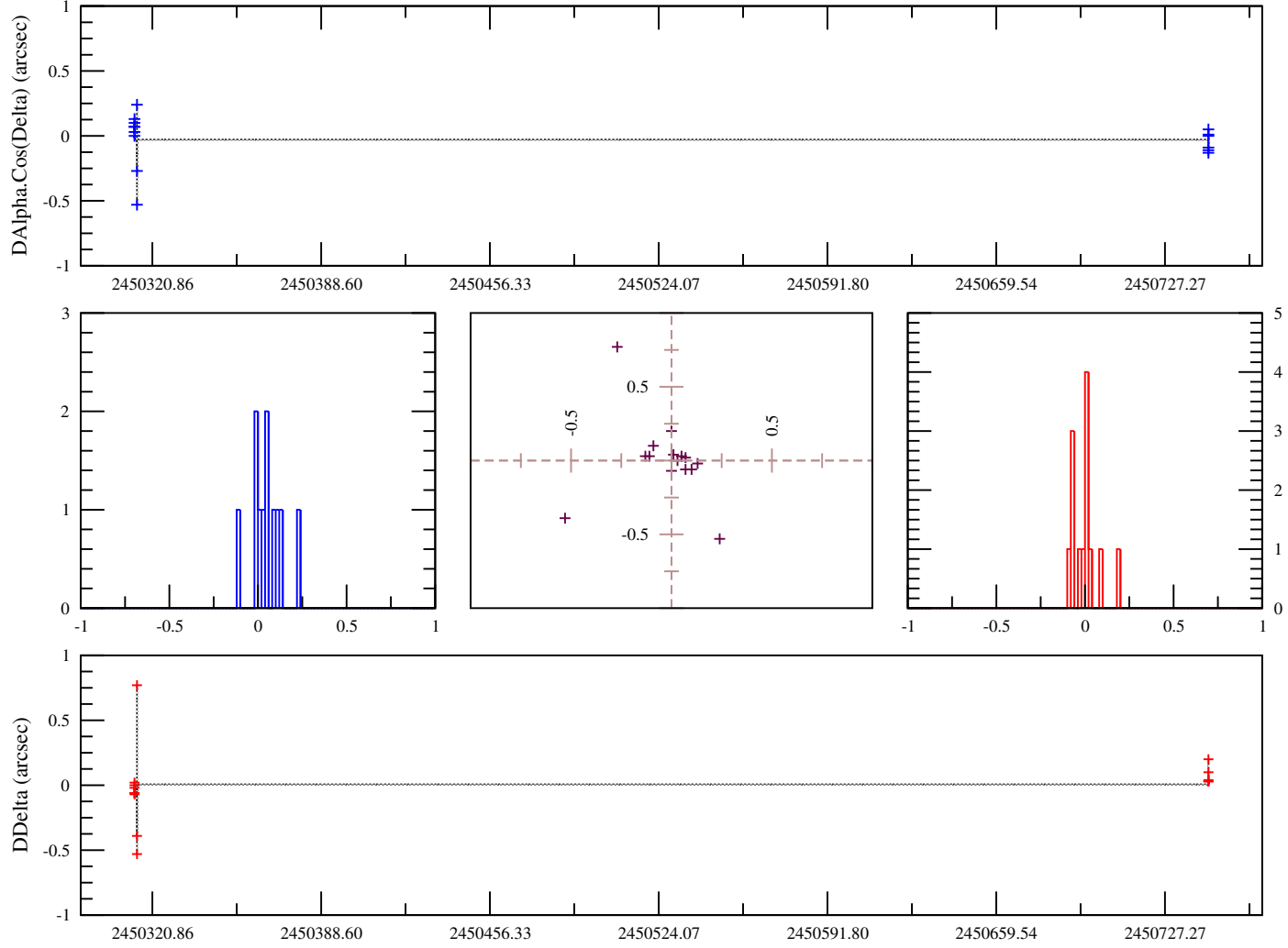
FIG. B.9: Observations Pascu D., 1996, USNO-Flagstaff, USA. OmC sur les observations de Thébé calculés avec l'éphéméride du JPL
