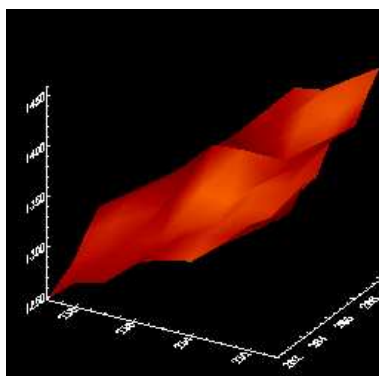
FIG. 2.5: L'image représente une zone de quelques pixels de l'image du TIM du Pic du Midi de la figure 2.4 par le logiciel TASPE. Il apparaît au centre le satellite Thébé.
