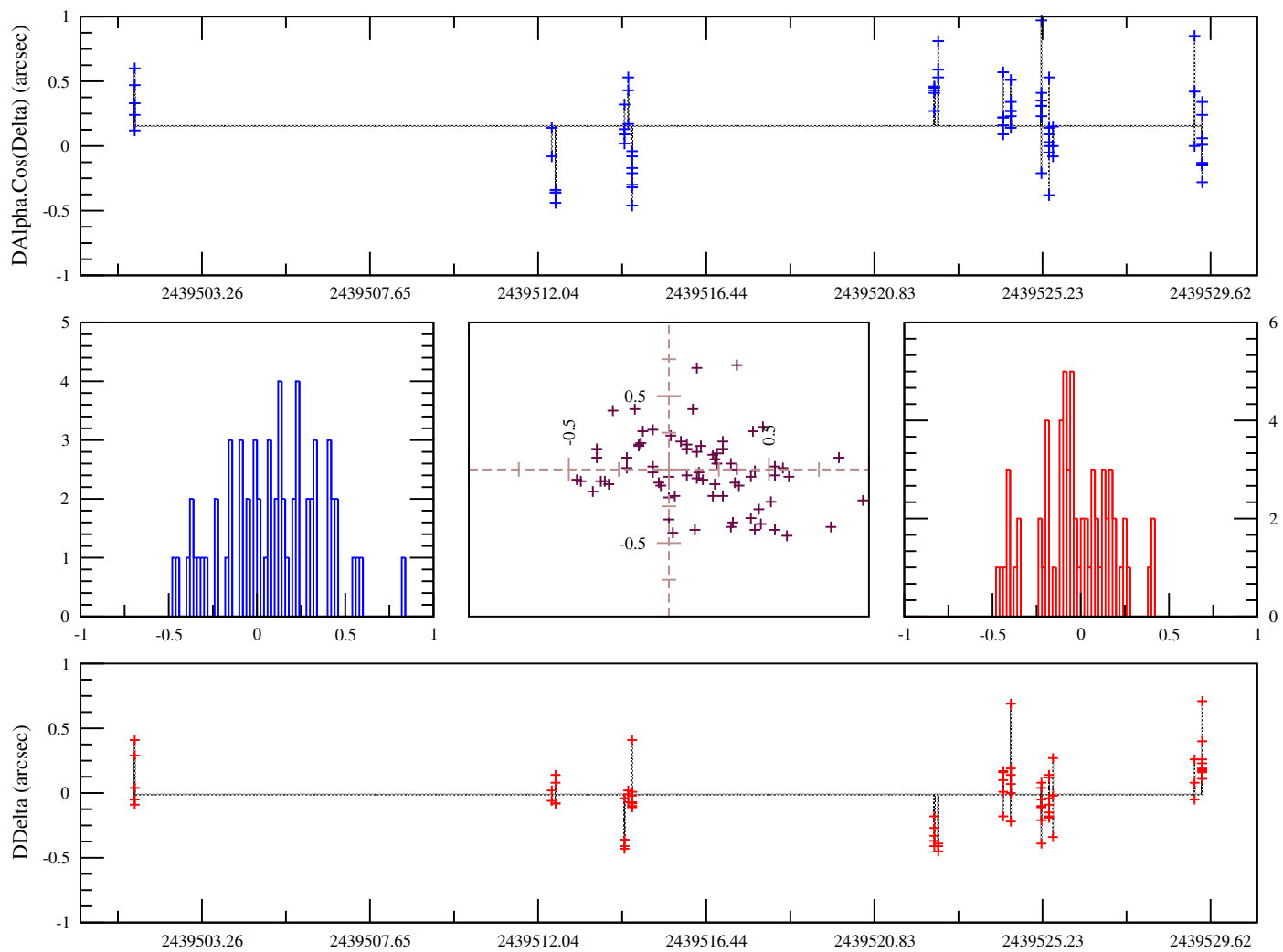
FIG. B.26: Observations Sudbury P.V., 1969, Obs. Kottomia, Egypte. OmC sur les observations d'Amalthée calculés avec l'éphéméride du JPL
