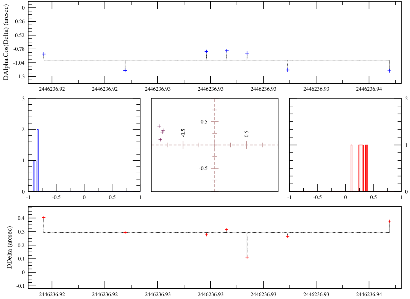
FIG. B.7: Observations Pascu D., 1985, USNO-Flagstaff, USA. OmC sur les observations de Thébé calculés avec l'éphéméride NJO2004A
