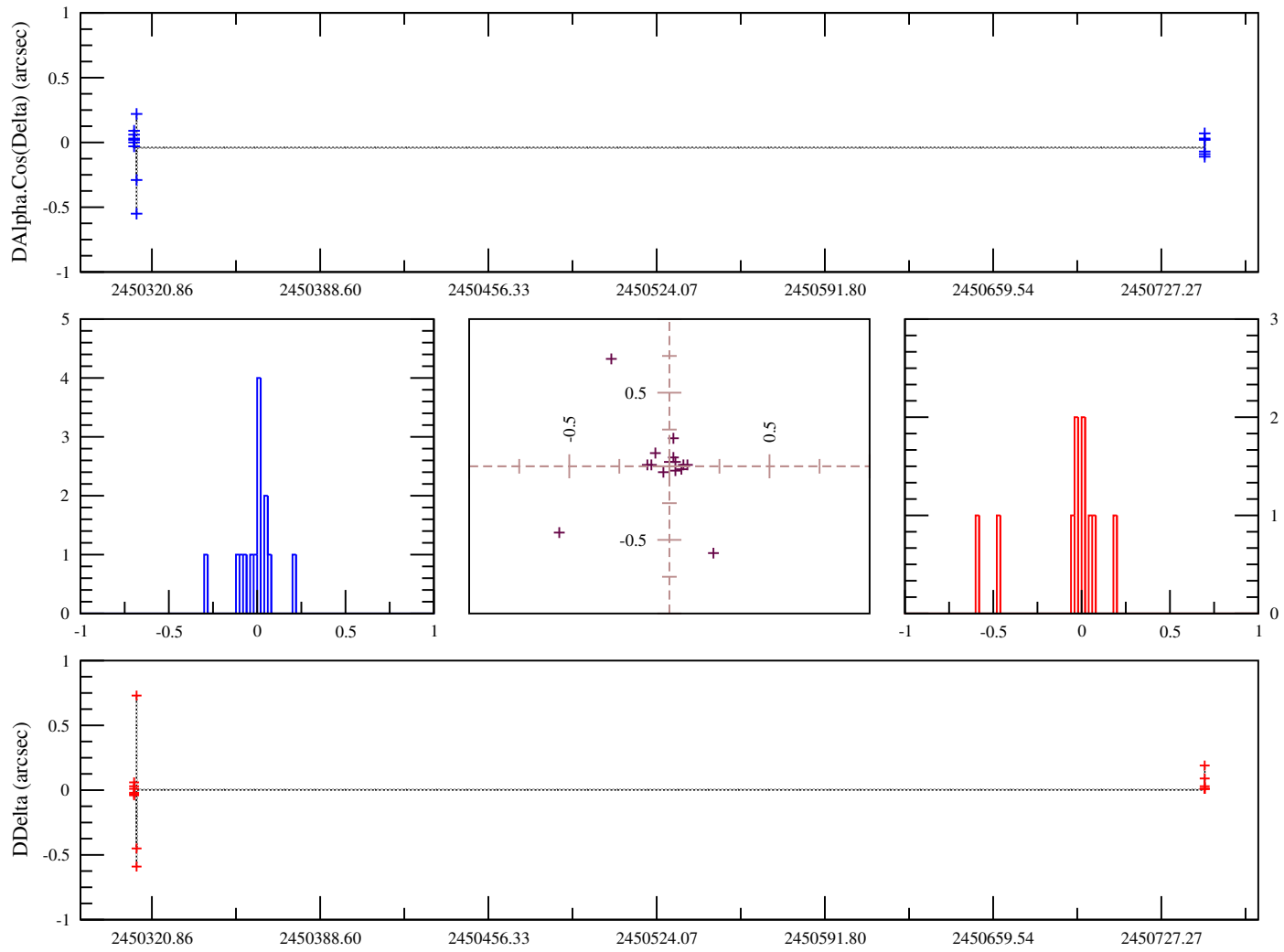
FIG. B.10: Observations Pasco D., 1996, USNO-Flagstaff, USA. OmC sur les observations de Thébé calculés avec l'éphéméride du JPL
