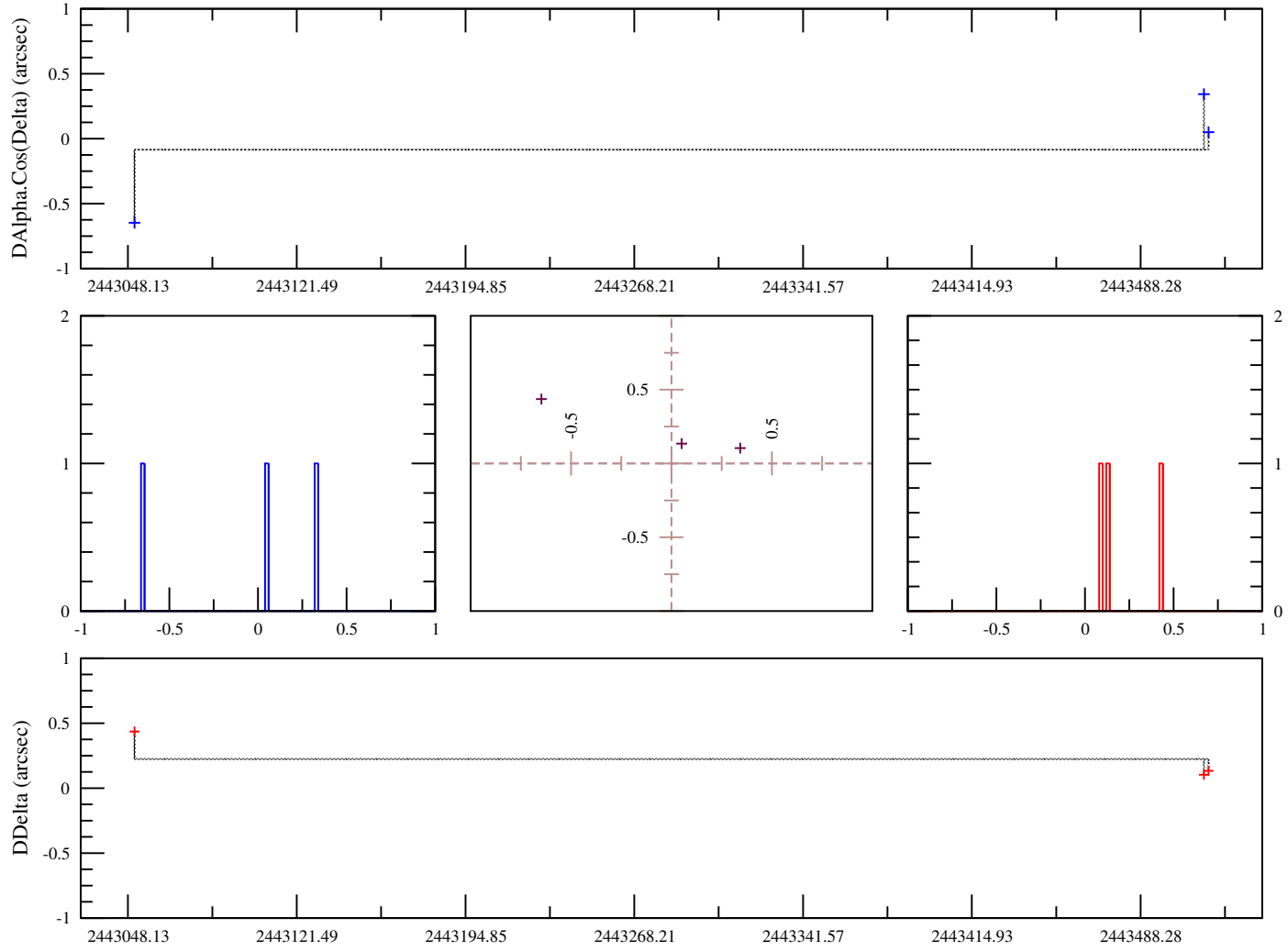
FIG. B.27: Observations Mulholland, 1977, Obs. McDonald, USA. OmC sur les observations d'Amalthee calculés avec l'éphéméride NJO2004A
