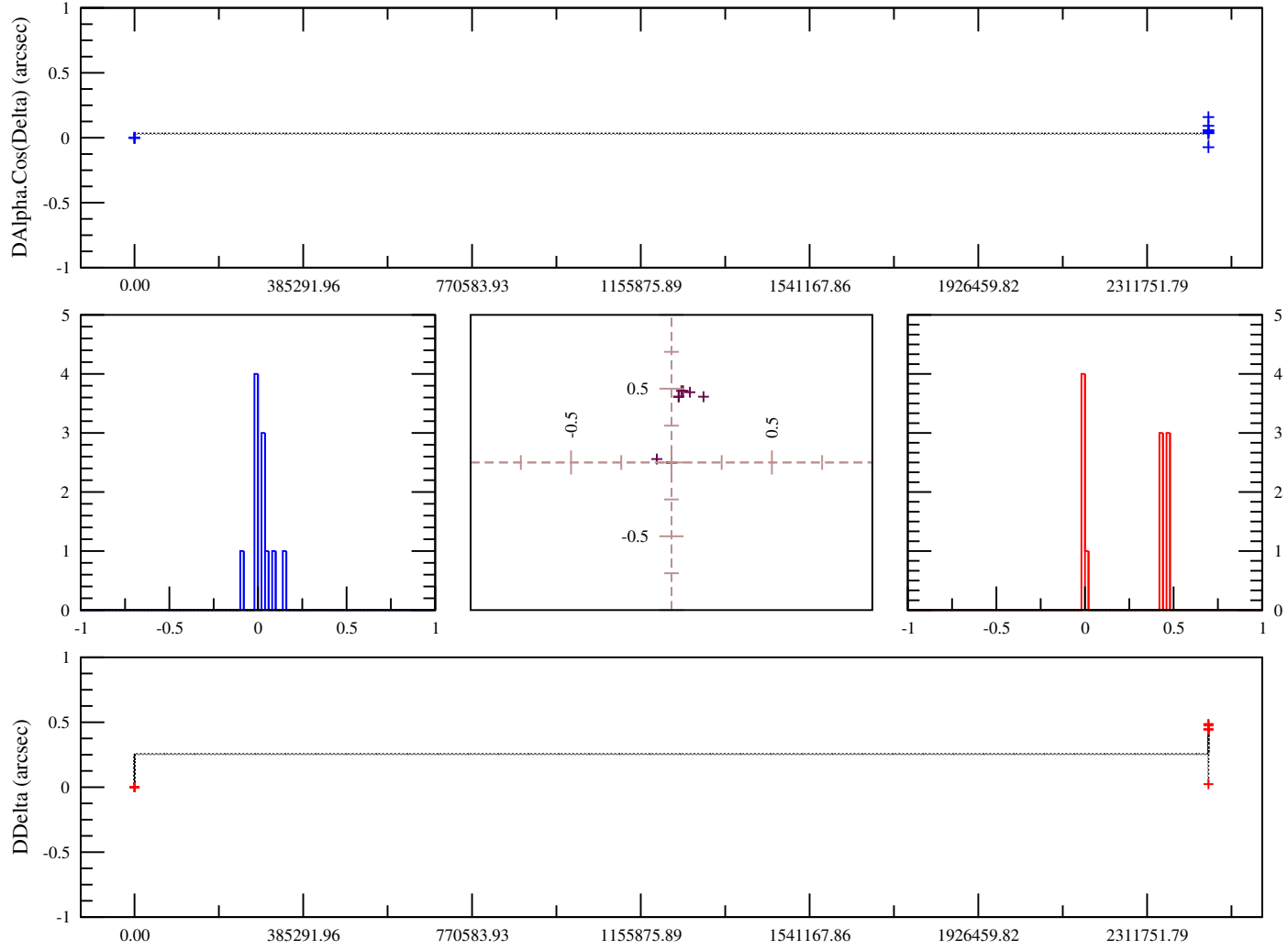
FIG. B.19: Observations Pascu D., Vachier F., 2000, USNO-Flagstaff, USA. OmC sur les observations d'Amalthée calculées avec l'éphéméride NJO2004A
