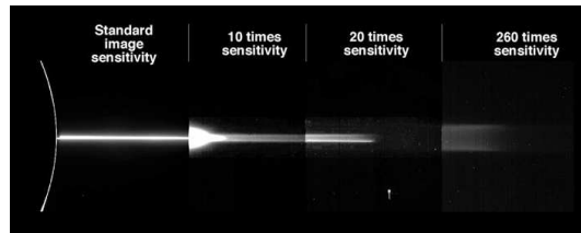
FIG. 1.5: Les anneaux de Jupiter vus par la sonde Galileo.
