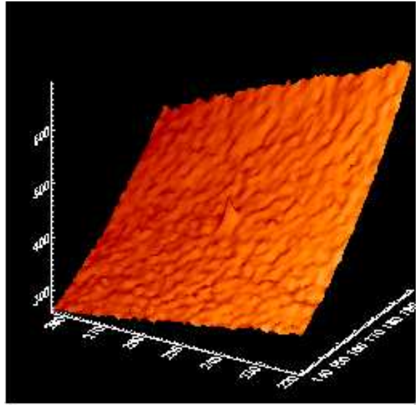
FIG. 2.7: On peut voir sur cette image le fort gradient de lumière émise par Jupiter, le bruit de mesure ainsi qu'une étoile (au centre) dont le profil se situe légèrement au dessus du bruit.
