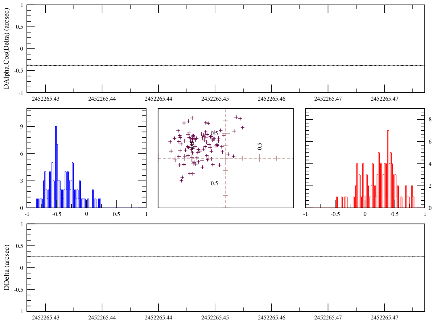
FIG. B.3: Observations Colas F., Vachier F., 2001, Pic du Midi, France. OmC sur les observations de Thébé calculés avec l'éphéméride NJO2004A
