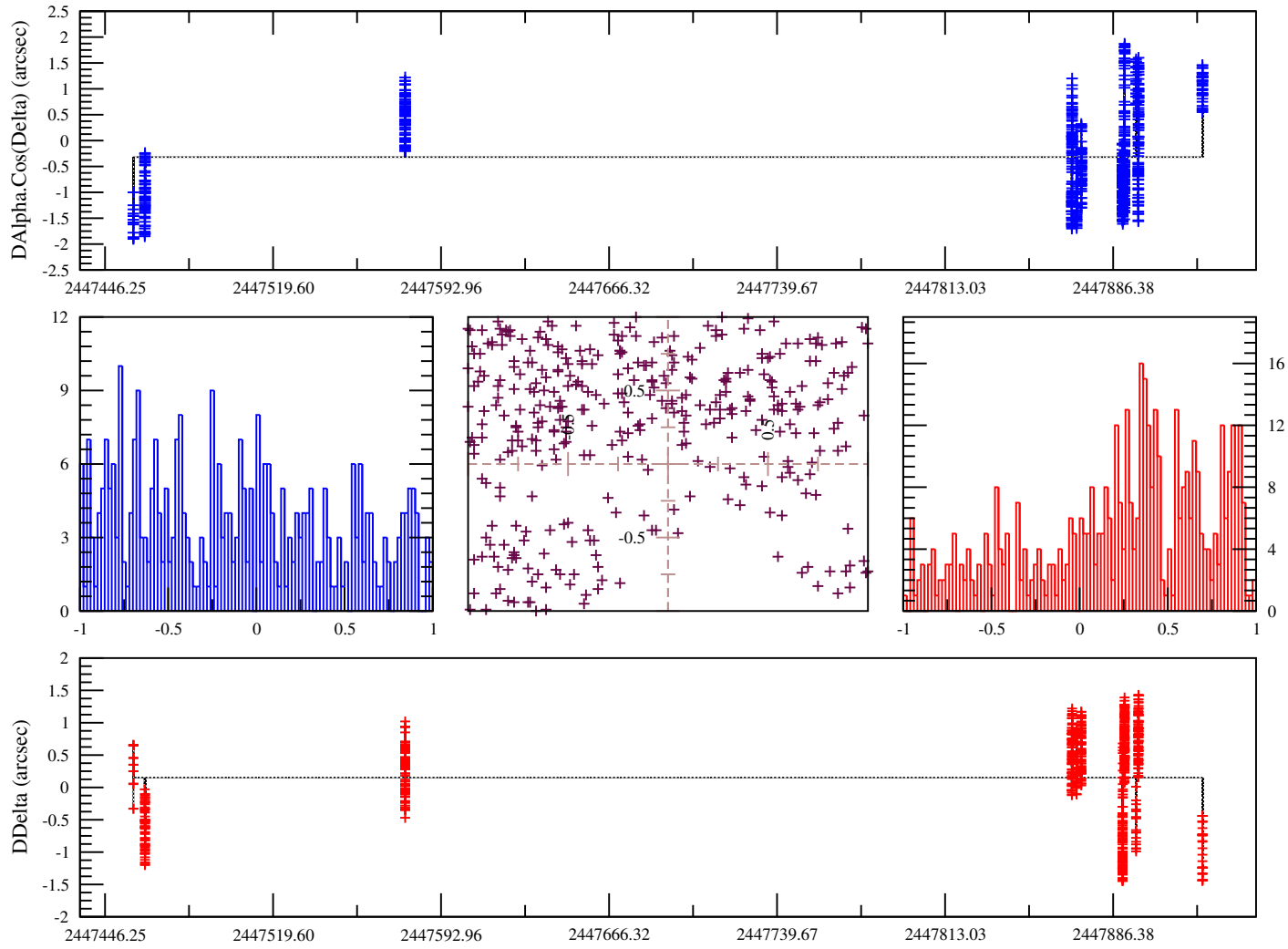
FIG. B.6: Observations Colas F., 1991, Pic du Midi, France. OmC sur les observations de Th e calcul es avec l' ph m ride du JPL
