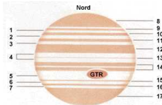
FIG. 1.3: Description des bandes à la surface de Jupiter.
