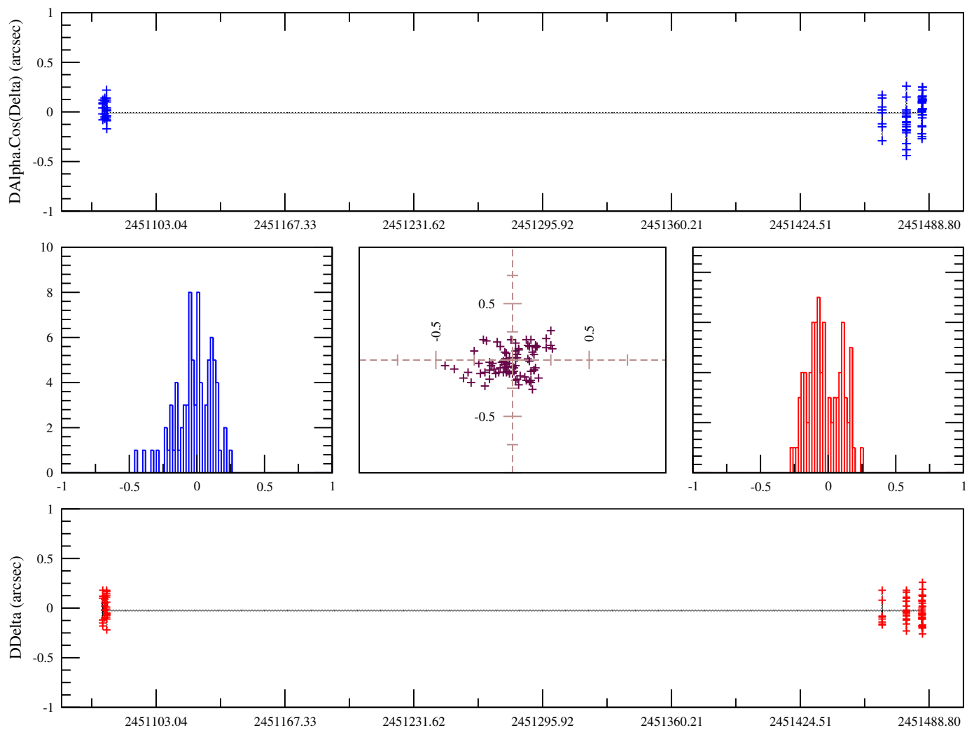
FIG. B.14: Observations Kulyk et al., 1998-2000, Pik Terskol, Ukraine. OmC sur les observations de Thébé calculées avec l'éphéméride du JPL
