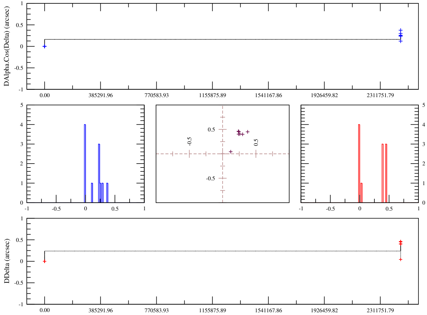
FIG. B.20: Observations Pasco D., Vachier F., 2000, USNO-Flagstaff, USA. OmC sur les observations d'Amalthée calculés avec l'éphéméride du JPL
