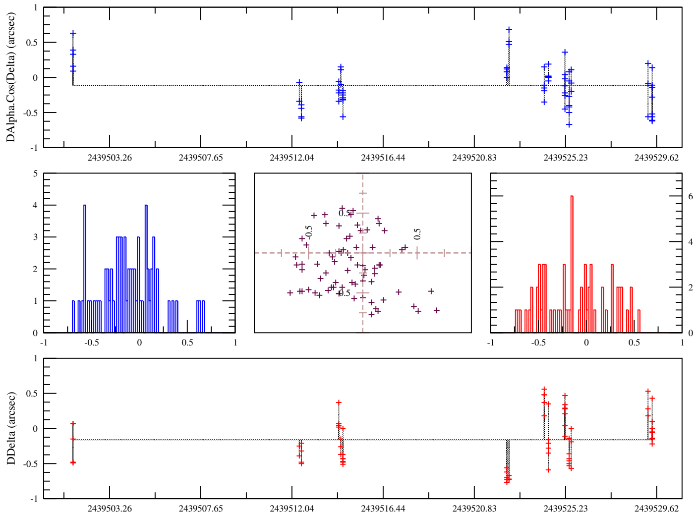
FIG. B.25: Observations Sudbury P.V., 1969, Obs. Kottomia, Egypte. OmC sur les observations d'Amalthée calculés avec l'éphéméride NJO2004A
