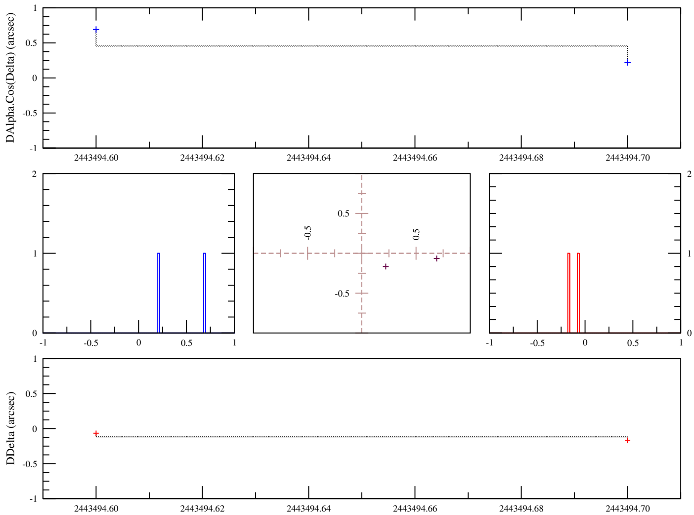
FIG. B.23: Observations Ianna P. A., 1979, Mc Cormick, USA. OmC sur les observations d'Amalthée calculés avec l'éphéméride NJO2004A
