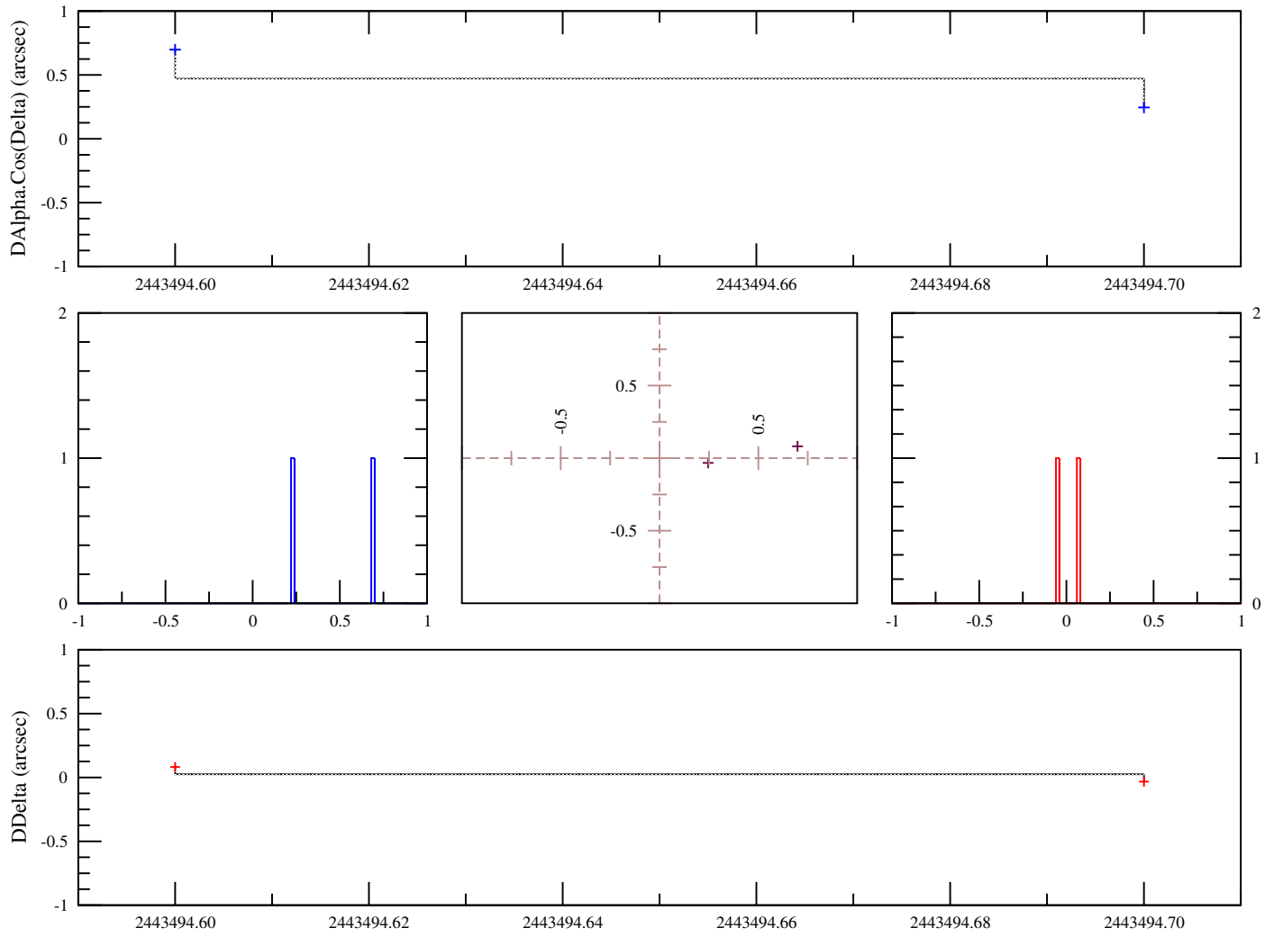
FIG. B.24: Observations Ianna P.A., 1979, Mc Cormick, USA. OmC sur les observations d'Amalthée calculés avec l'éphéméride du JPL
