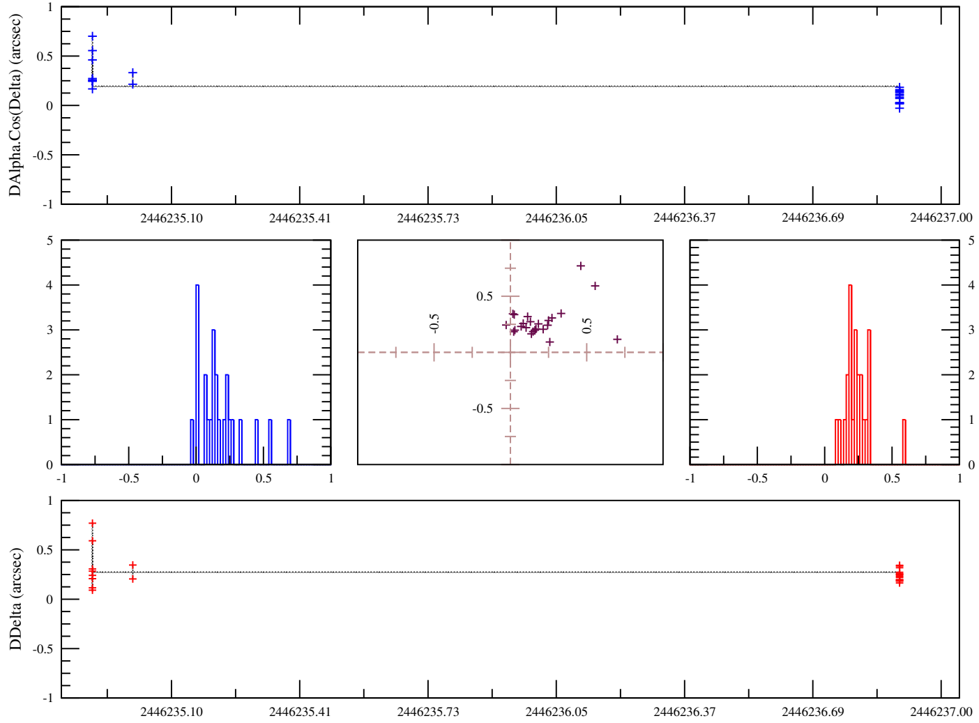
FIG. B.21: Observations Pascu D., 1985, USNO-Flagstaff, USA. OmC sur les observations d'Amalthée calculés avec l'éphéméride NJO2004A
