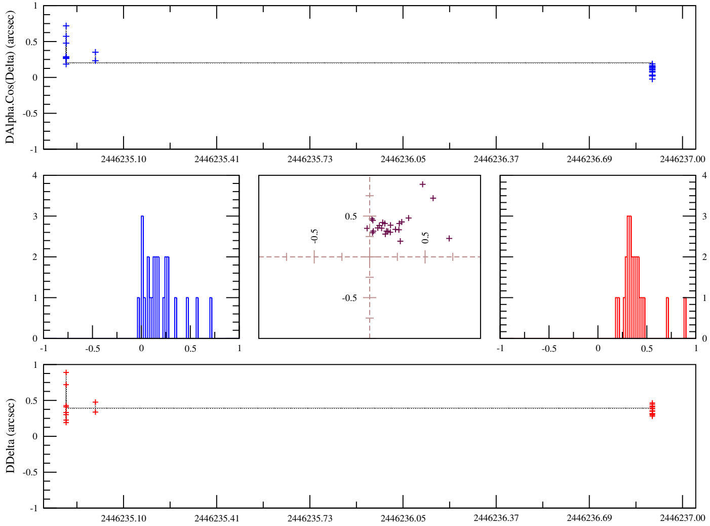
FIG. B.22: Observations Pasco D., 1985, USNO-Flagstaff, USA. OmC sur les observations d'Amalthee calculés avec l'éphéméride du JPL
