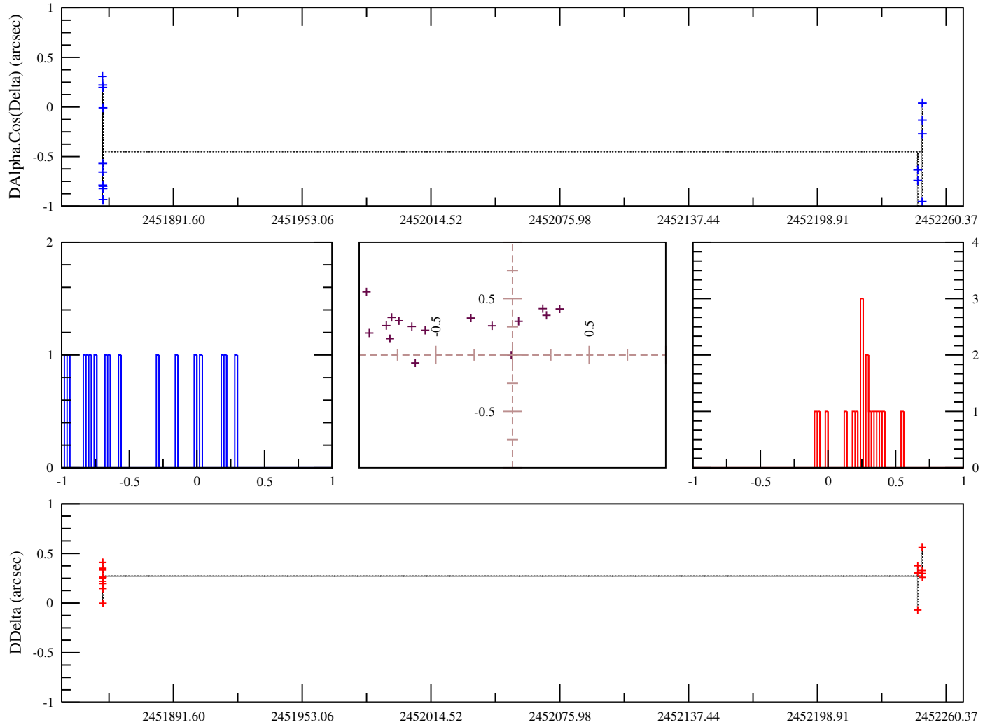
FIG. B.12: Observations Pasco D., Vachier F., 2001, USNO-Flagstaff, USA. OMC sur les observations de Thébé calculées avec l'éphéméride du JPL
