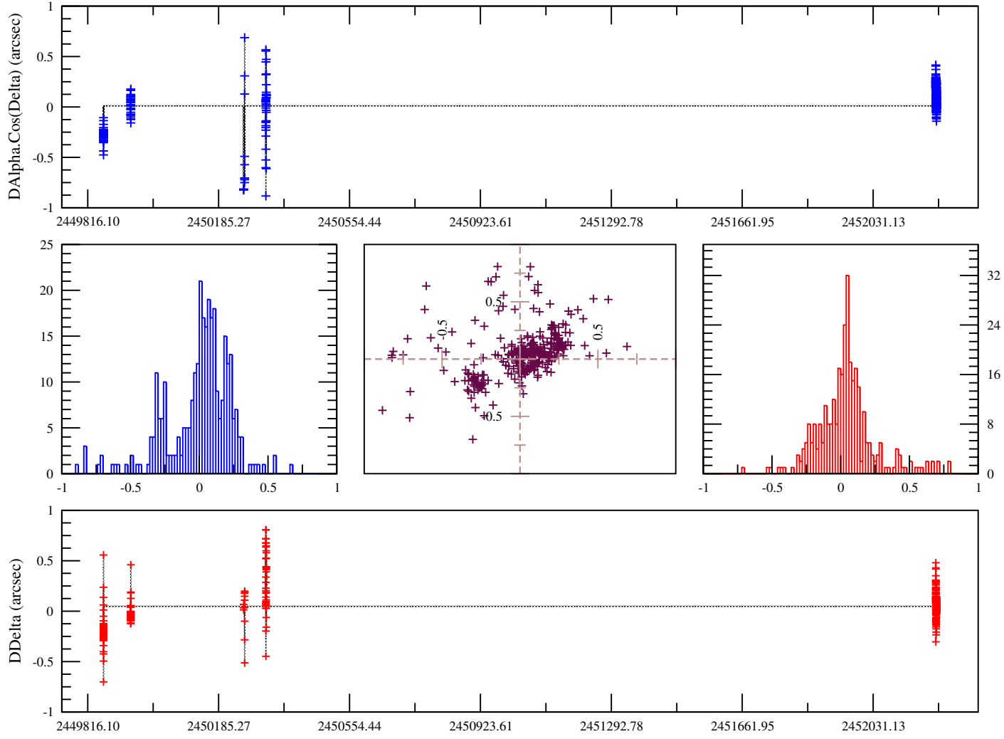
FIG. B.1: Observations Veiga C., Vieira-Martins R., 1995-2001, LNA Itajuba Brasil. OmC sur les observations de Thébé calculés avec l'éphéméride NJO2004A
