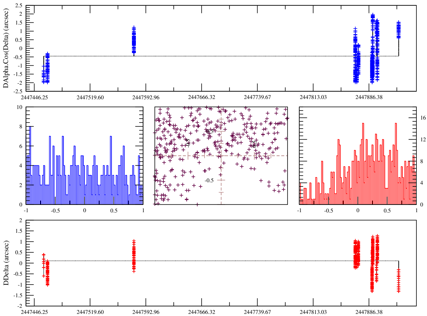
FIG. B.5: Observations Colas F., 1991, Pic du Midi, France. OmC sur les observations de Th b  calcul es avec l' ph m ride NJO2004A
