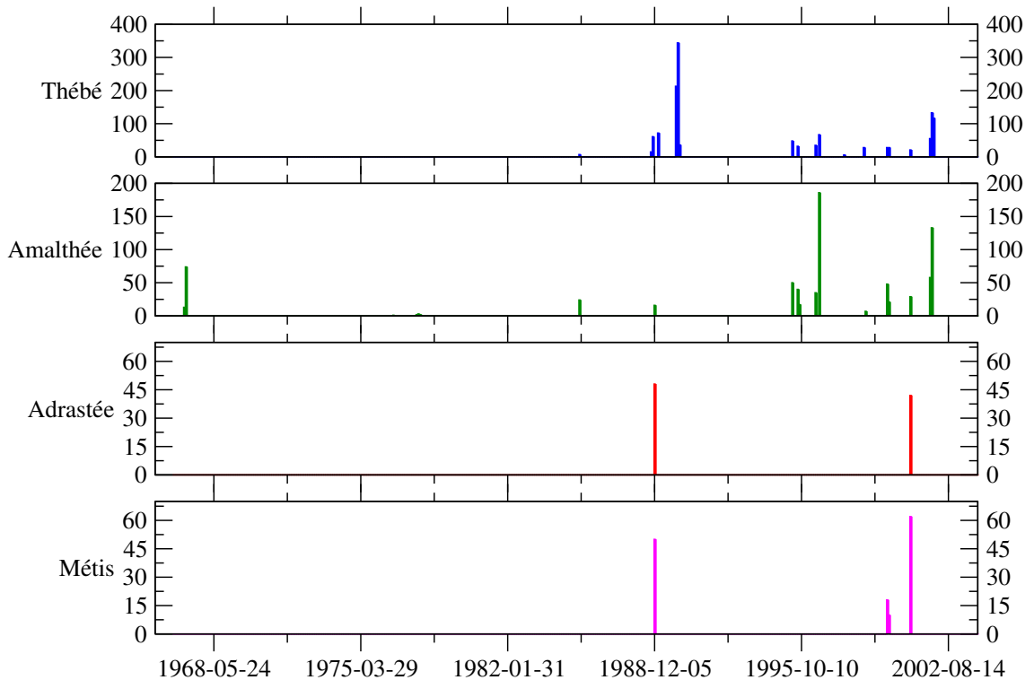
FIG. 2.9: Chronogrammes des observations disponibles, des quatre satellites internes de Jupiter. Ils caractérisent la répartition des observations, de 1968 à 2003. Les échelles en Y pour chaque satellite, sont différentes. Elles représentent le nombre d'observation faites dans le mois.
