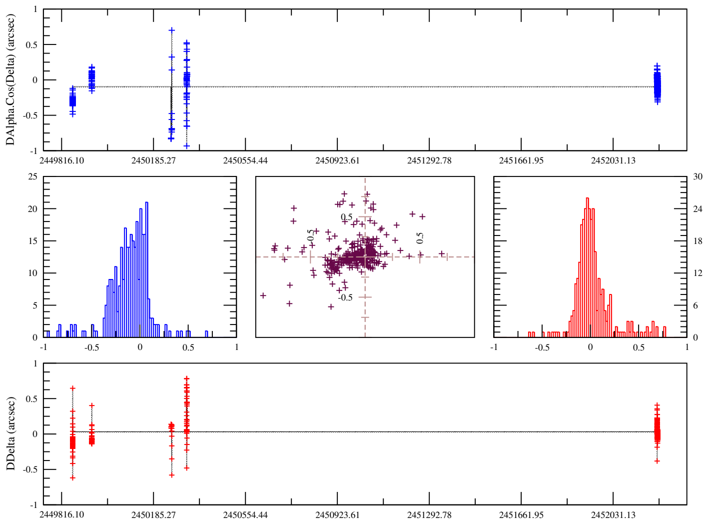
Observations Veiga C., Vieira-Martins R., 1995-2001, LNA Itajuba, Brasil. [UAI=874] Satellite Thébé - JPL Ephemeris
