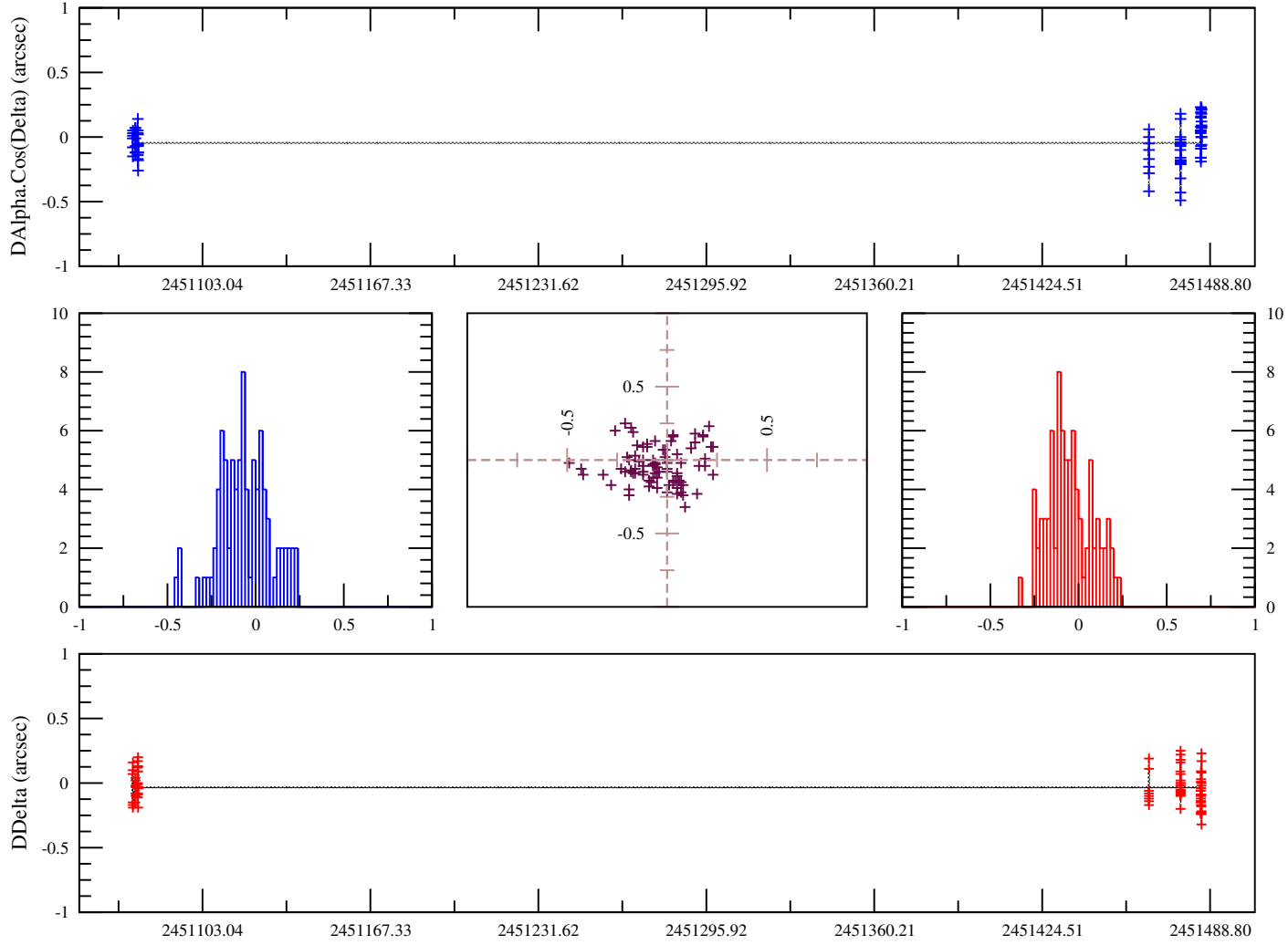
FIG. B.13: Observations Kulyk et al., 1998-2000, Pik Terskol, Ukraine. OmC sur les observations de Thébé calculés avec l'éphéméride du JPL
