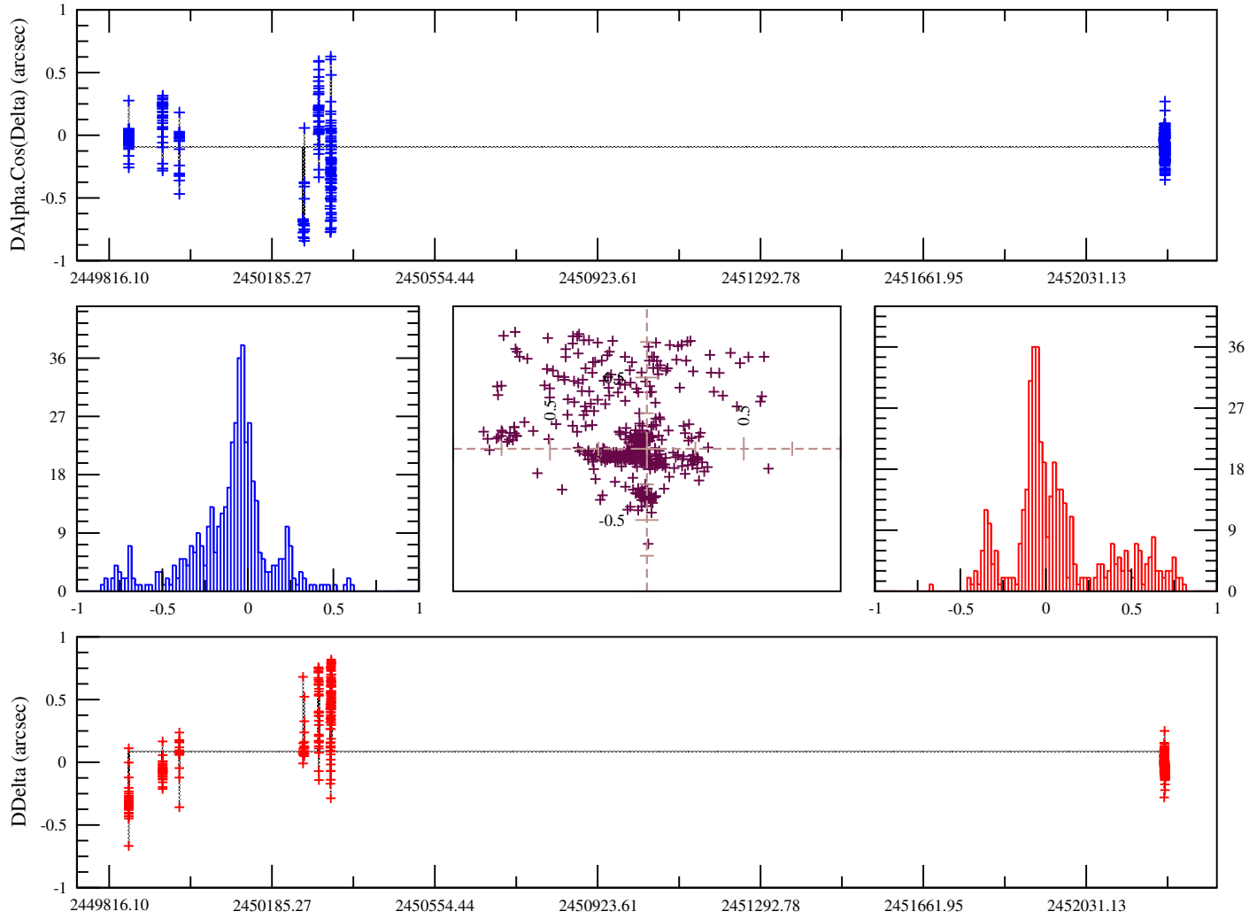
FIG. B.16: Observations Veiga C., Vieira-Martins R., 1995-2001, LNA Itajuba Brasil. OmC sur les observations d'Amalthée calculés avec l'éphéméride du JPL
